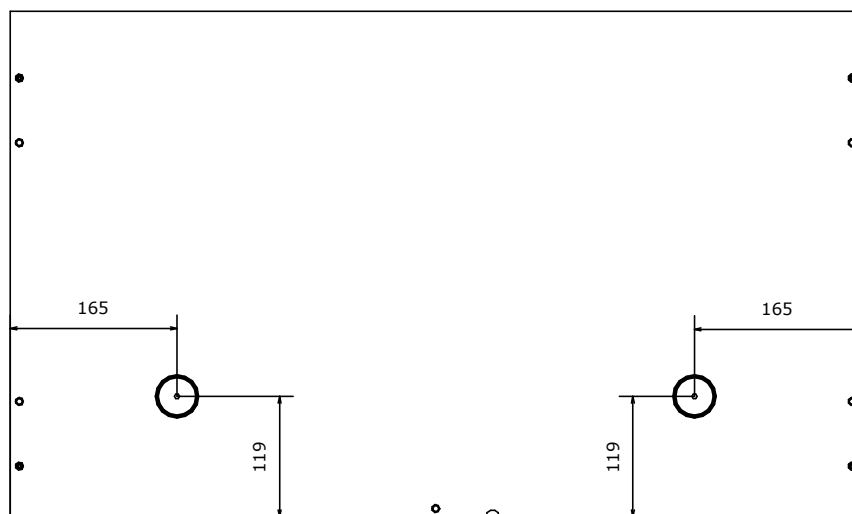
Деталь комода №1 Нелицевая сторона
