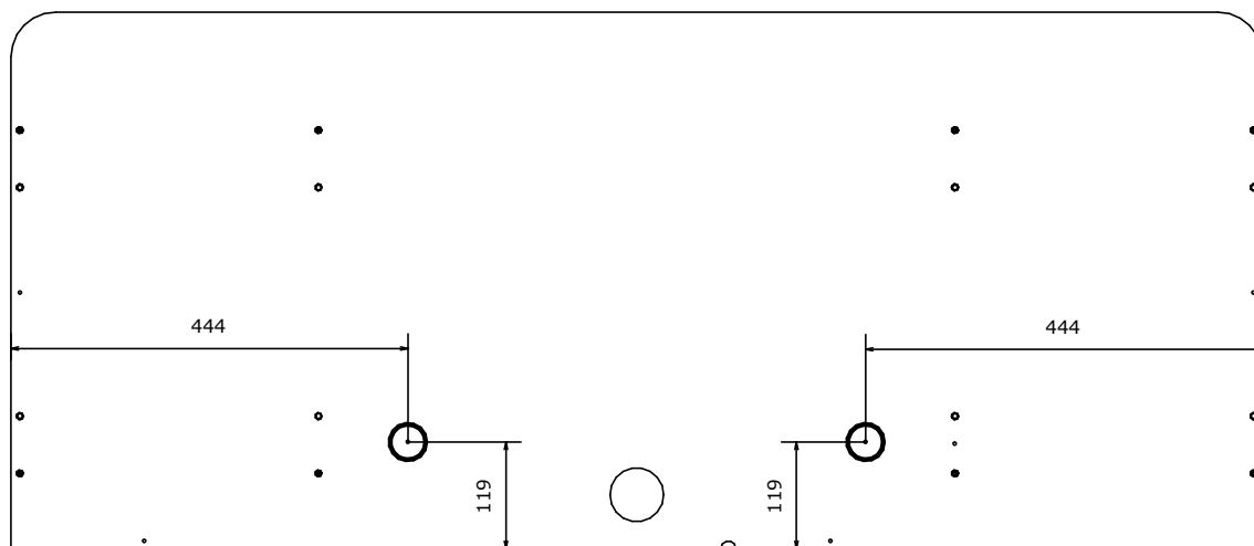
Деталь стола №3 Не лицевая сторона
