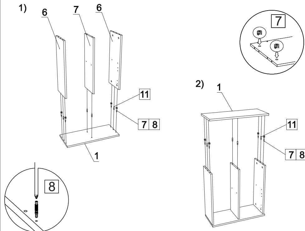
Сборка полки
